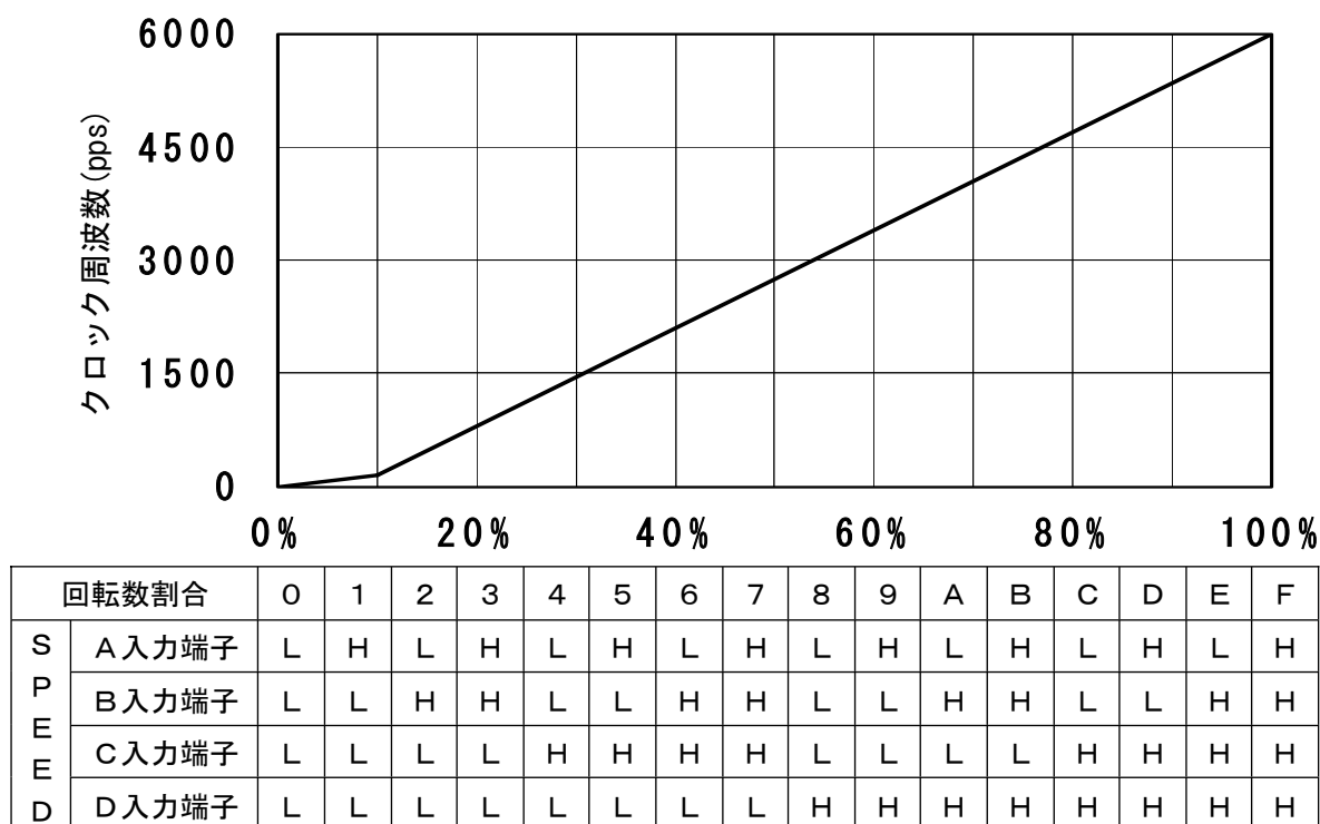
第8図 HIGH SPEEDポリウムを6kppsに調整した時の SPEED A～D 入力信号による回転数変化例
