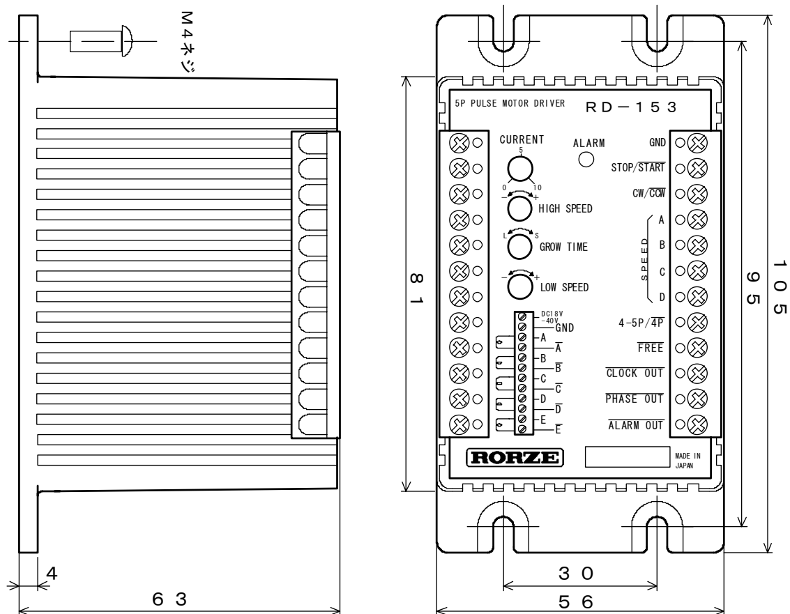
第16図 RD-153外形寸法図 単位 (mm)
