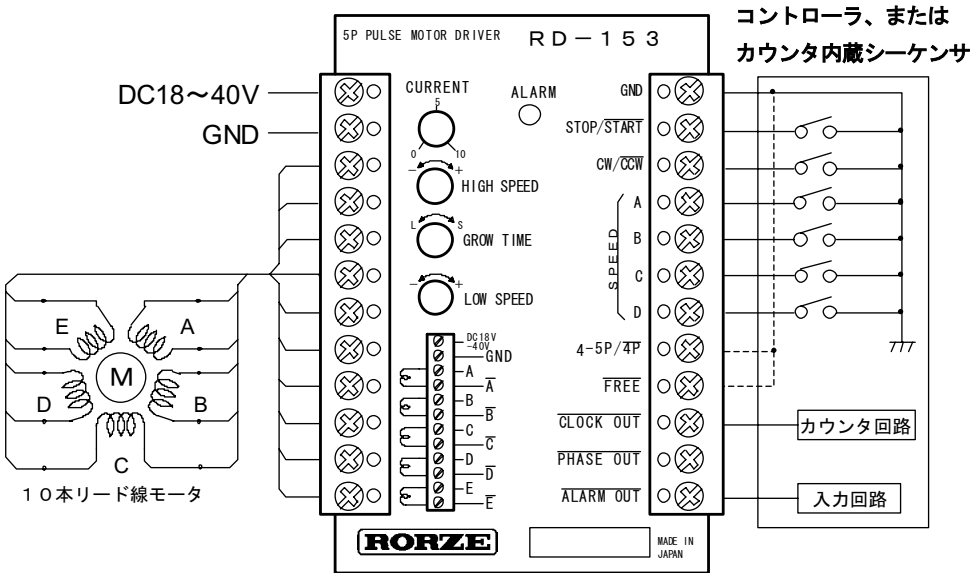
第 1 4 図 結線図
